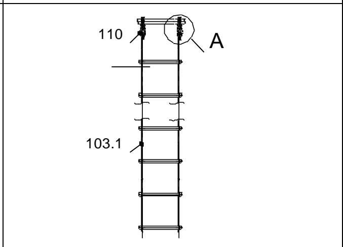
Поз.103 (для 01.21.8.06.490.03.06-14)
