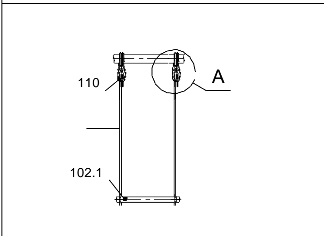
Поз.102 (для 01.21.8.06.490.03.06-24)
