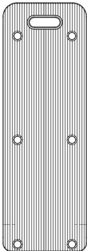
1 Боковая панель стеллажа X2
